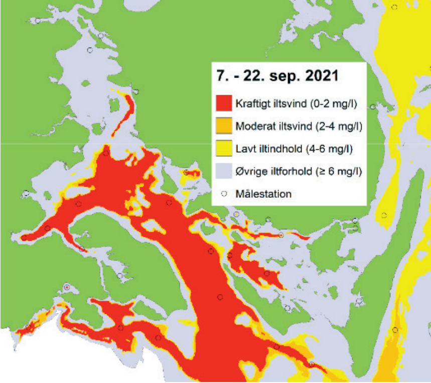
Auf der Karte des DCU zeigt die rote Farbe starken Sauerstoffmangel an. Die gelbe Farbe zeigt Bereiche, in denen niedrige Sauerstoffwerte gemessen wurden. Die Angaben beziehen sich auf den Zeitraum 7. bis 22. September.
