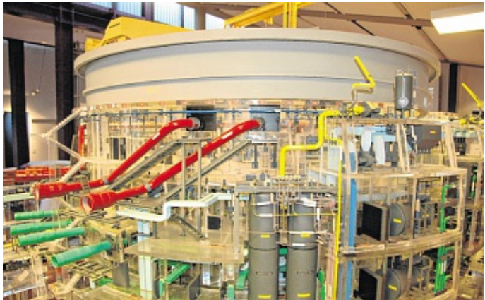
So sieht es hinter dem Beton der Reaktorkuppel aus. Das detailgetreue Modell im Maßstab 1:50 war vom Kraftwerksbetreiber einst zu Ausbildungszwecken erstellt worden. MEHMEL
